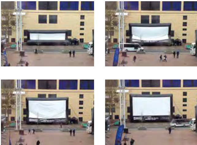
Aufstellen einer Leinwand 16m x 8m innerhalb weniger Minuten durch die Kraft eines leistungsstarken Gebläses
